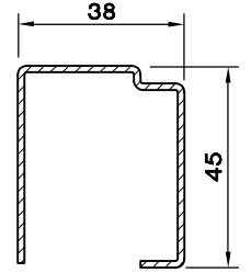
KANAT-74 DESTEK SAÇI (1.5) 5153.411
