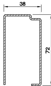
KAPI -100 DESTEK SAÇI (1.5) 5153.511
