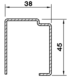
KANAT-74 DELİKLİ DESTEK SAÇI (1.5) 5253.411
