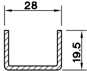
U PROFİLİ (2.0) 5199.111
