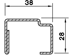
KANAT-56 DESTEK SAÇI (1.5) 5153.231
