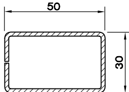
KUTU PR. (30 X 50 X 2.0) 5399.222
