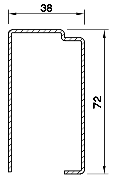
KAPI -100 DELİKLİ DESTEK SAÇI (1.5) 5253.511
