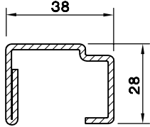
KANAT-56 DESTEK SAÇI (2.0) 5153.232
