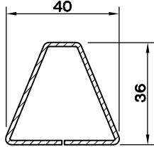
135° KÖŞE DÖNÜŞ DESTEK SAÇI (1.5) 5399.421
