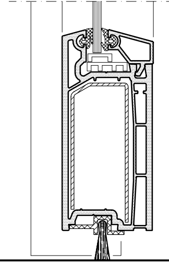
KESİT
