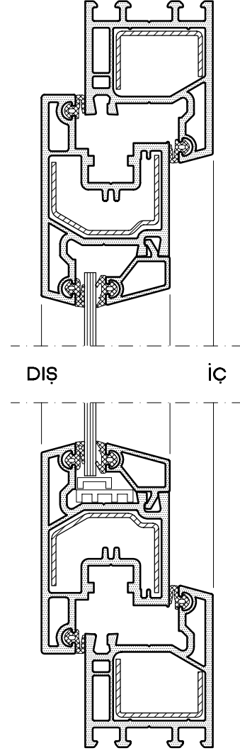
KESİT
