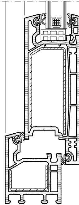
KESİT
