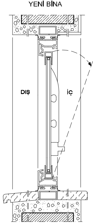
KESİT
