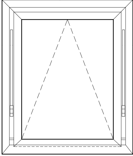
İÇ GÖRÜNÜŞ
