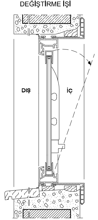
KESİT
